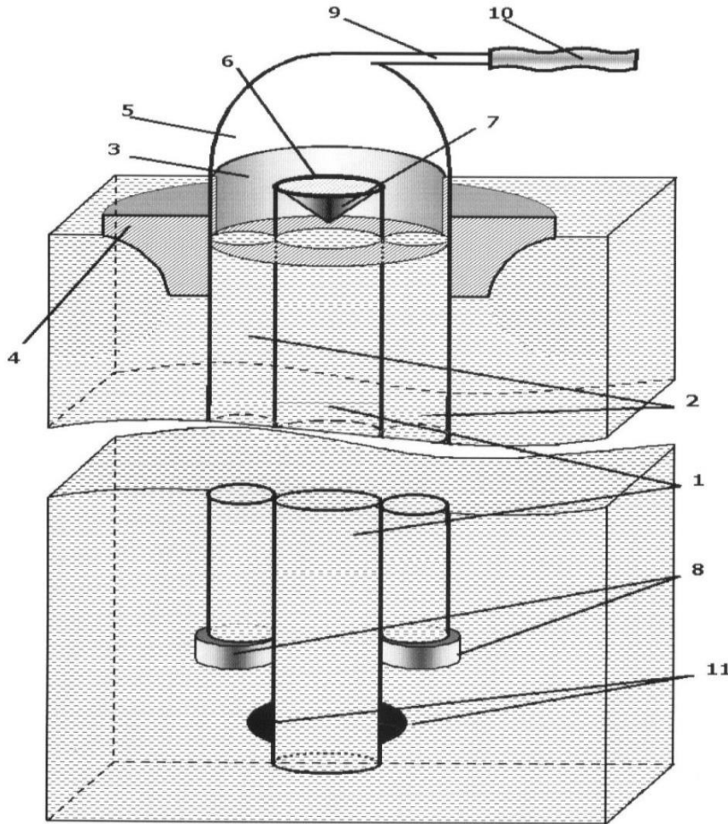
ნახ. 2.10. სიღრმისეული წყლებიდან ზედაპირზე აირთა ნარევის ამოსატანი დანადგარი.
