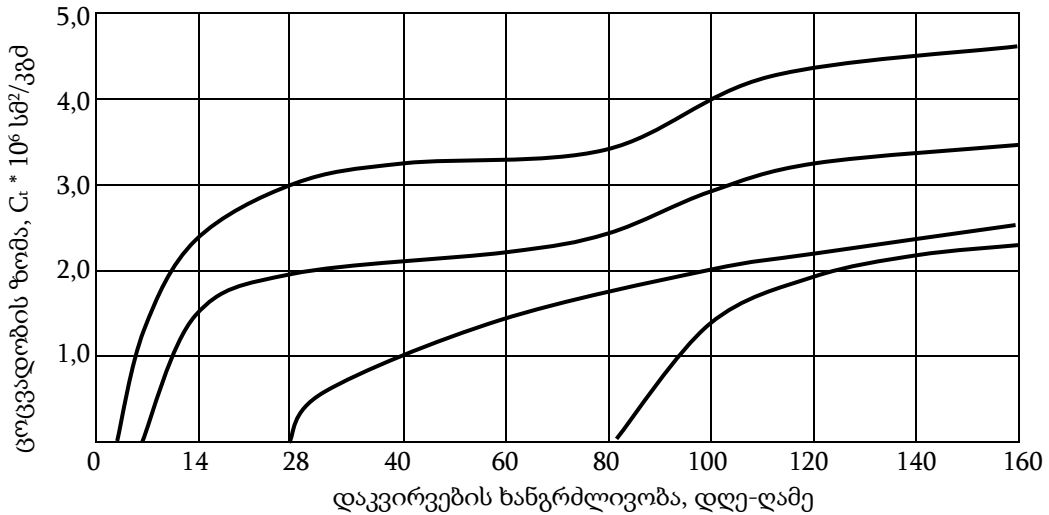
ნახ.1.2.გ. ცოცვადობის ზომა ბეტონისათვის მარკით, M600
