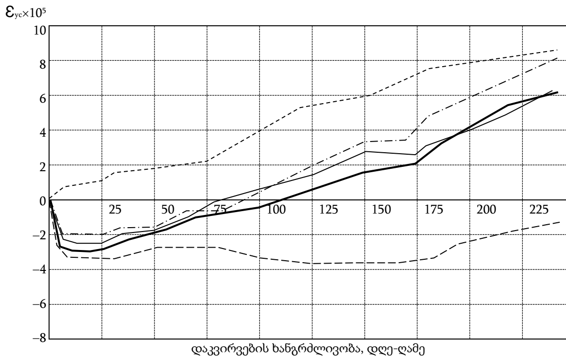
ნახ.4.15. ნარჩენი დეფორმაციები ღერძული გაჭიმვისას, 0,6R_{m} ; 5კ სერია
