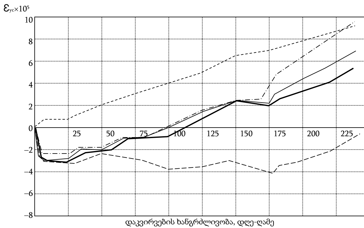
ნახ.4.14. ნარჩენი დეფორმაციები ღერძული გაჭიმვისას, 0,6R_{m} ; 4კ სერია
