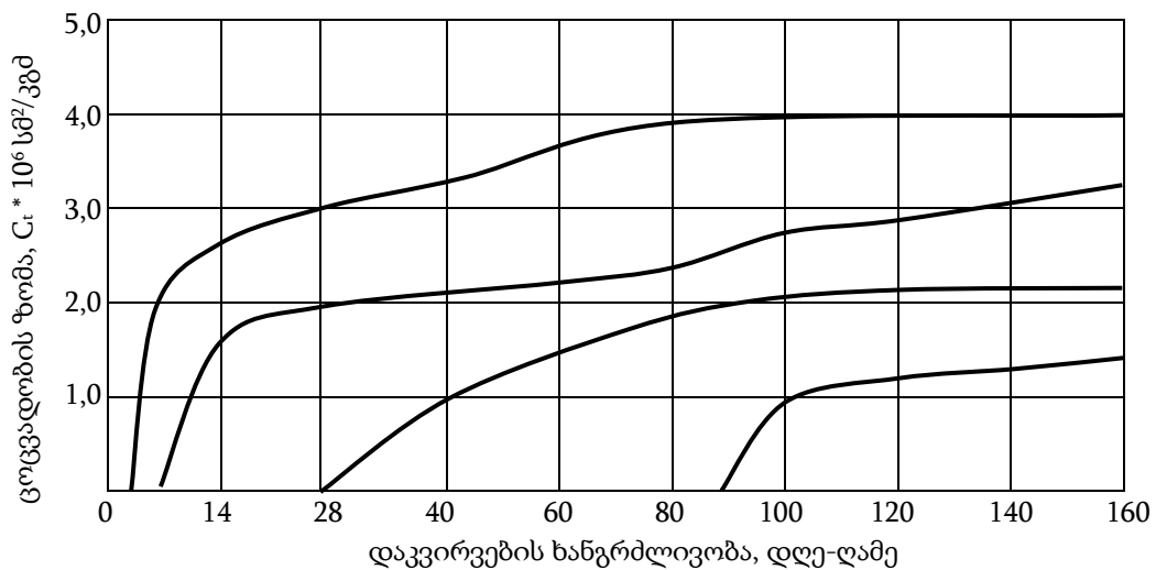
ნახ.1.2.ბ. ცოცვადობის ზომა ბეტონისათვის მარკით, M800
